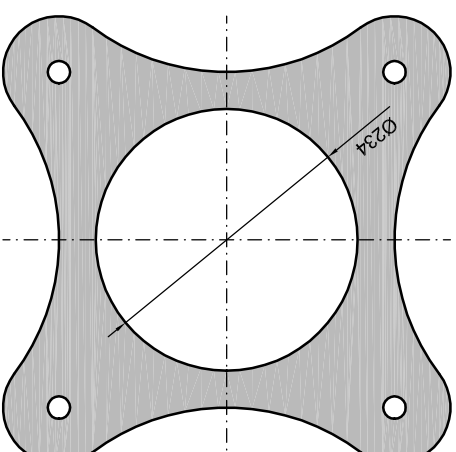
bovenaanzicht tussenplaat
