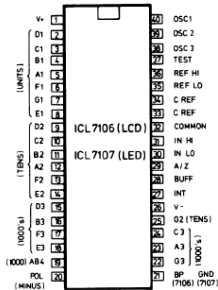
07 A/D-converter 3½ digit
