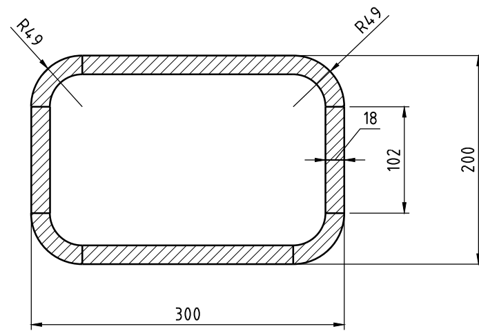
Doorsnede
