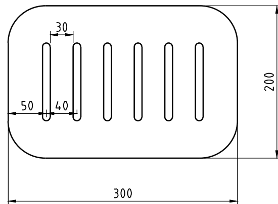
Vooraanzicht
