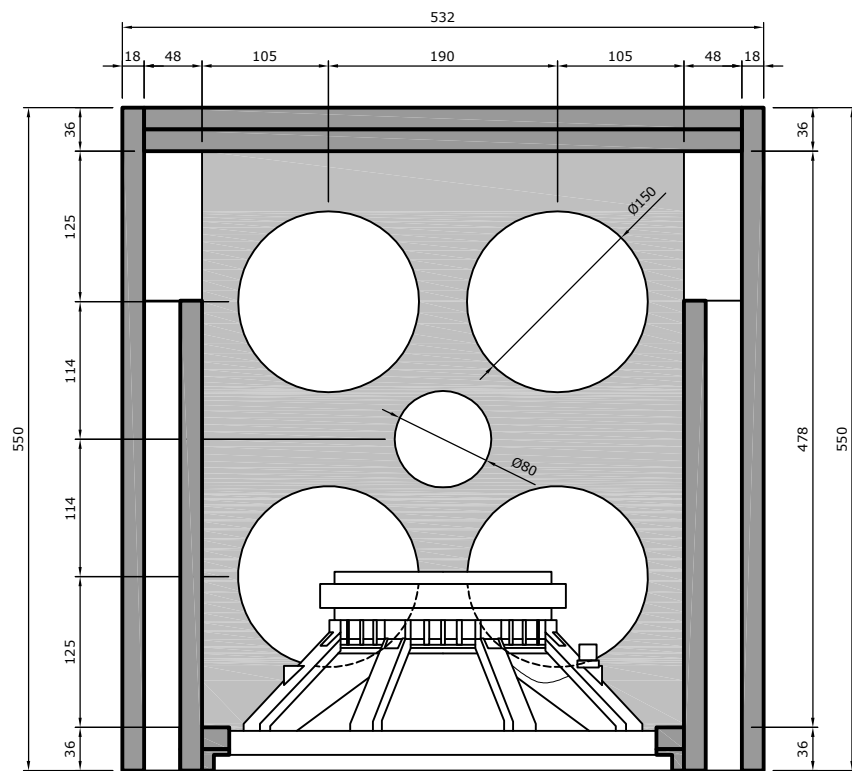
horizontale doorsnede
