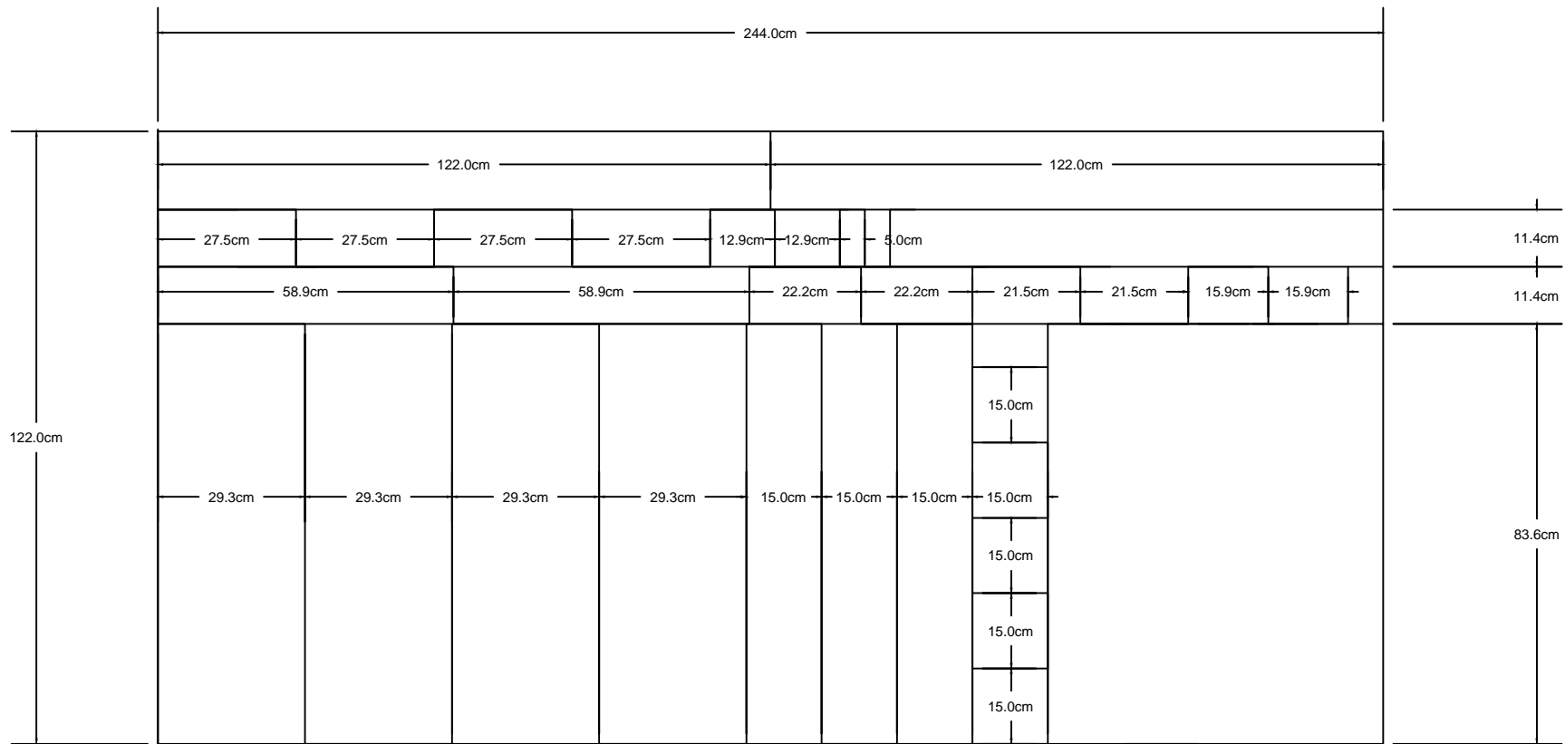
Zaagplan: Hans Materiaal: 18mm MDF
