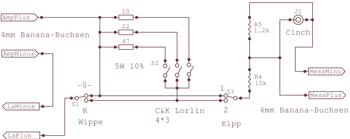
Schaltplan DLSA-Messbox M2
