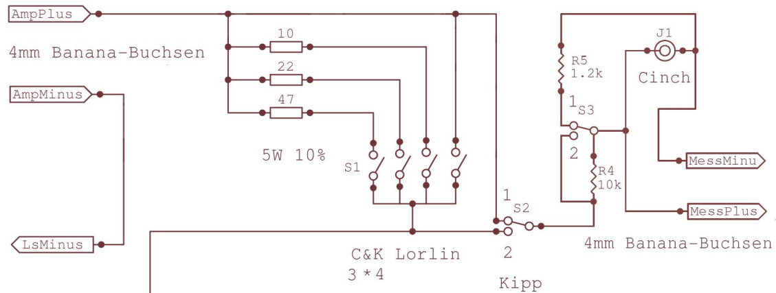
Schaltplan DLSA-Messbox M2
