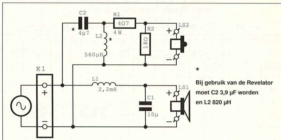
Figuur 2. Het uiterst simpele filter.
