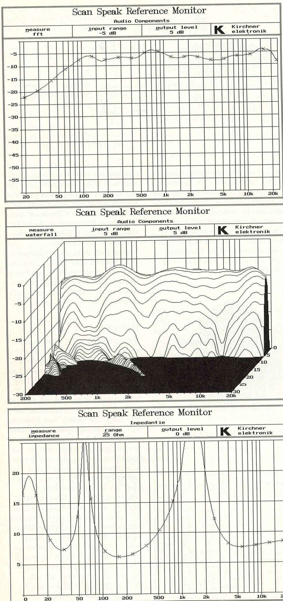
Figuur 5. De gebruikelijke metingen op een rijtje.
