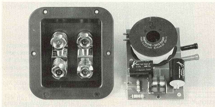
Figuur 3. Filter en aansluit-unit. Let op de montage van L1 en L2.
