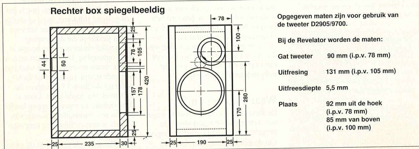
Figuur 1. Een simpel kastje dat snel te bouwen is. Let wel op de dikte van het materiaal.
