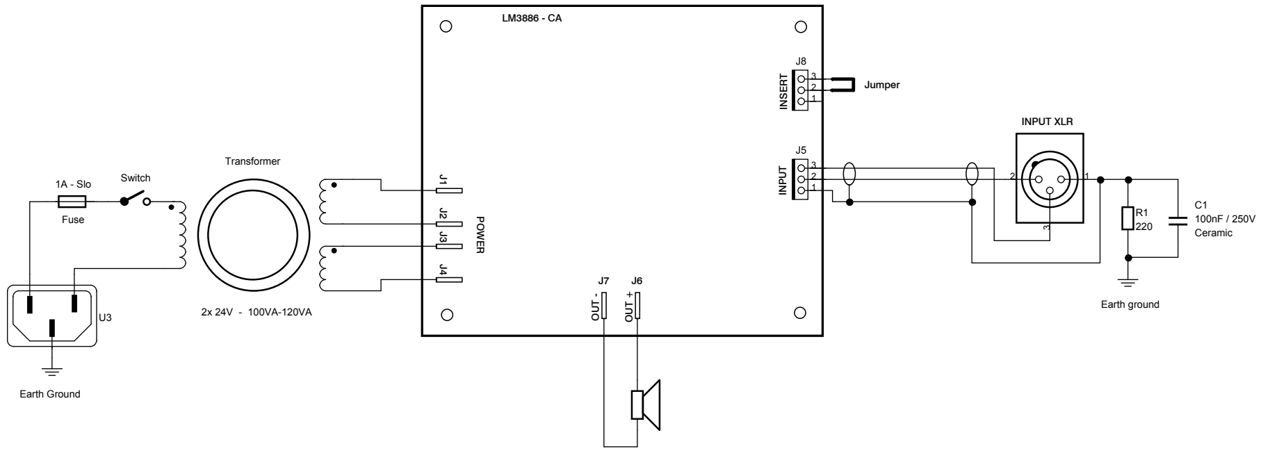
Aansluitschema Gebalanceerd
