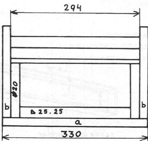
ACHTERAANZICHT.
