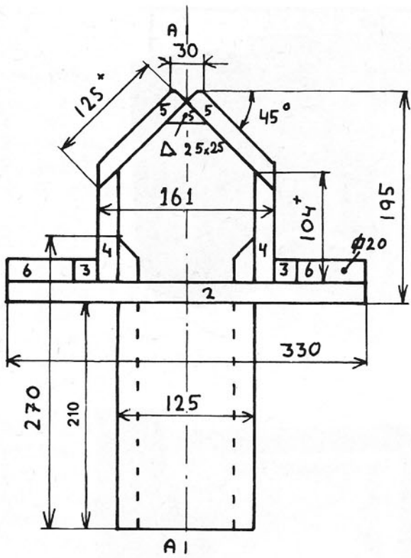
DOORSNEDE A-A
