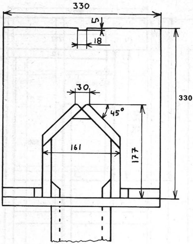
VOORAANZICHT
