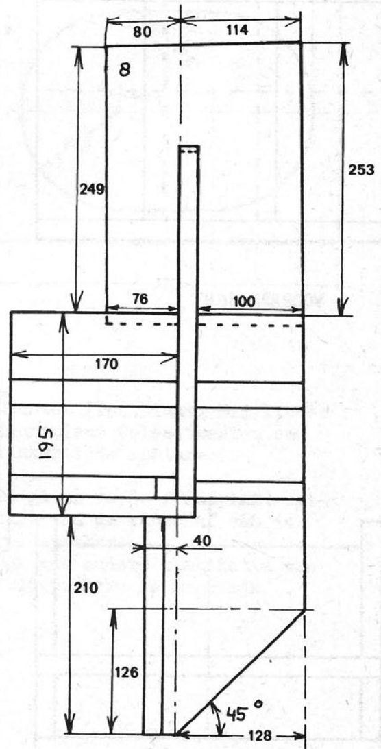
ZYAAANZICHT
