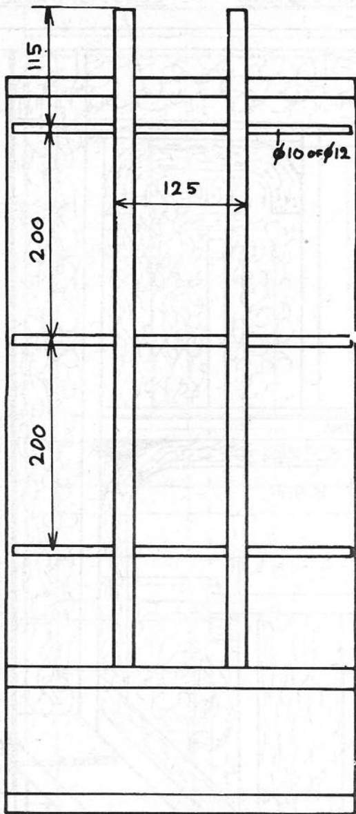
ACHTER AANZICHT
