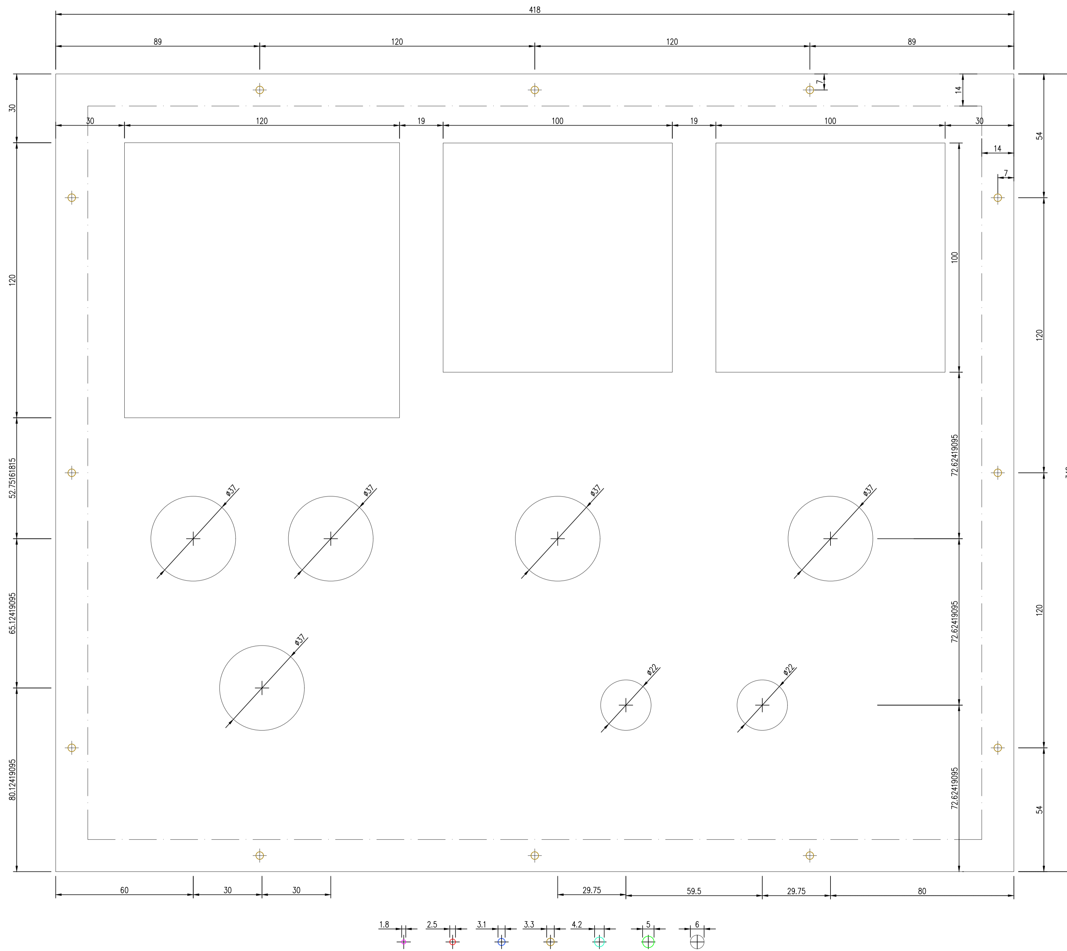
ROVFNAANZICHT CHASSIS
