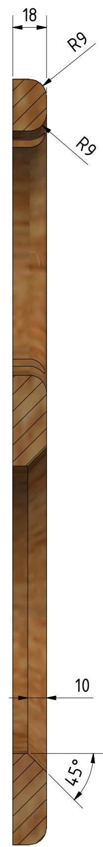
H-H ( 1 : 2 )
