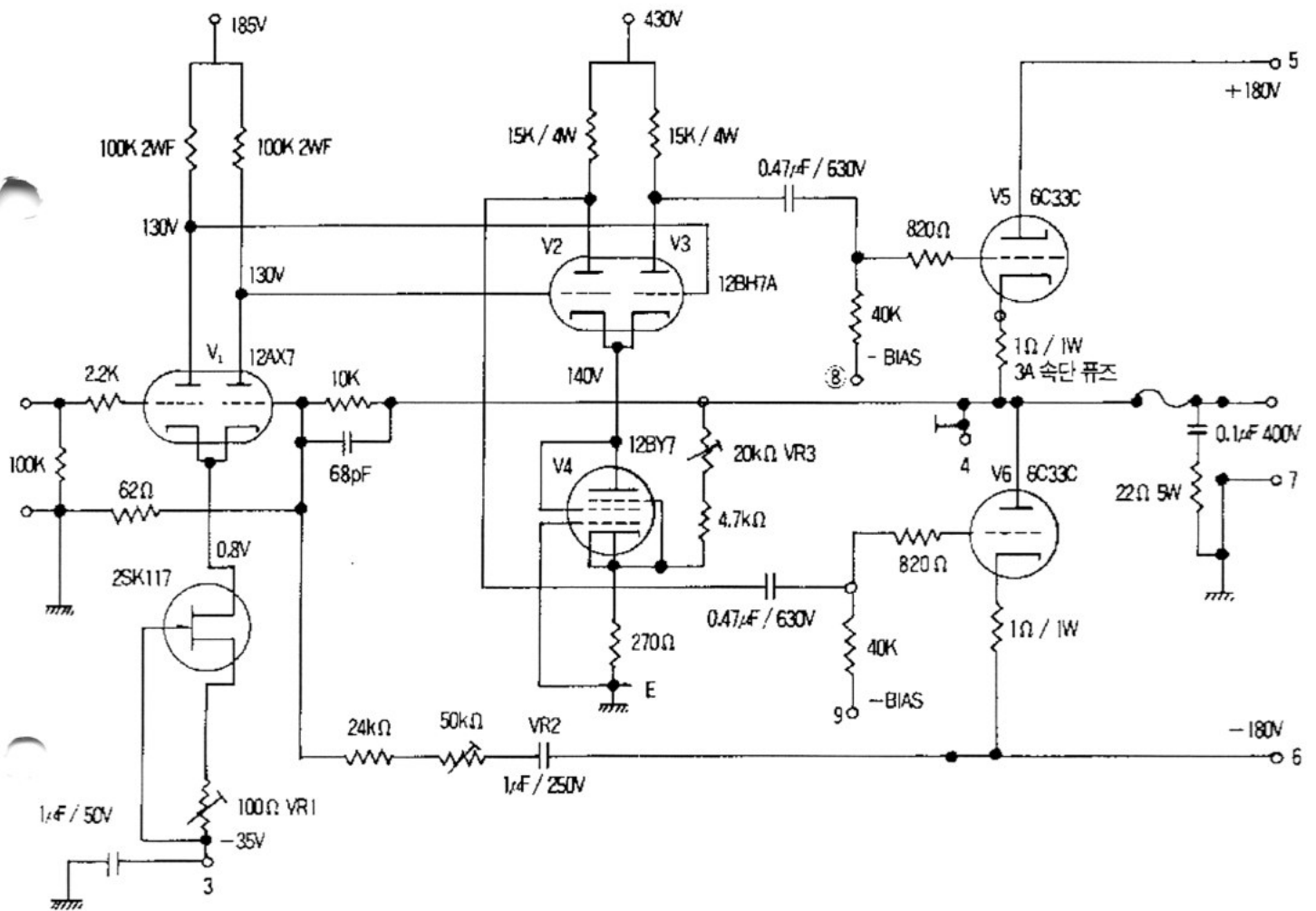
〈그림 3〉 6C33C OTL 파워 앰프 증폭부 회로도
