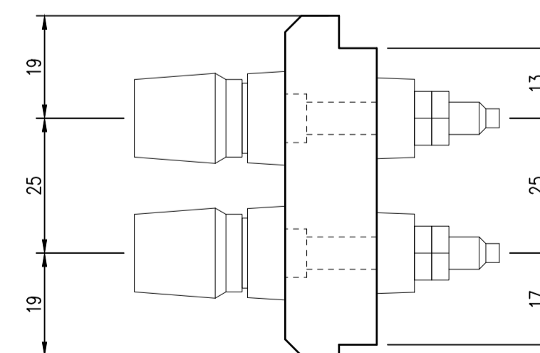
DOORSNEDE
