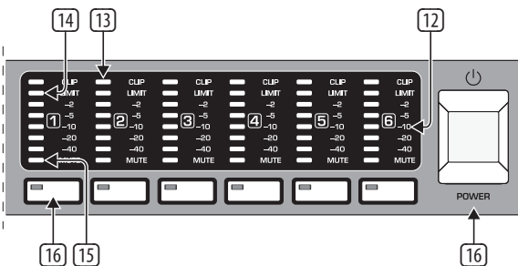
Afb. 2.3: Uitgang-LED's
