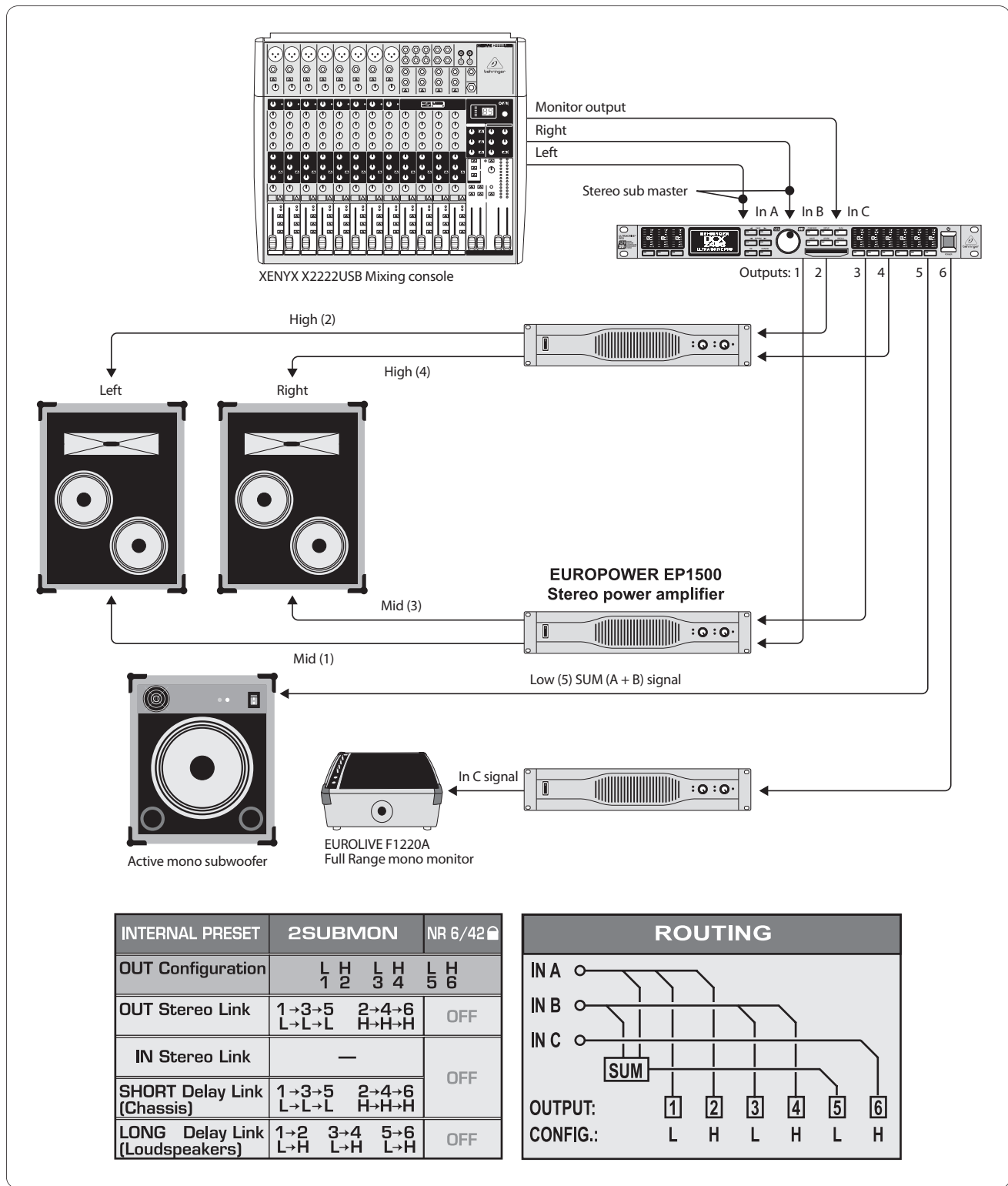
Afb. 6.6: Stereo 2-weg-gebruik plus subwoofer en extra monitor
