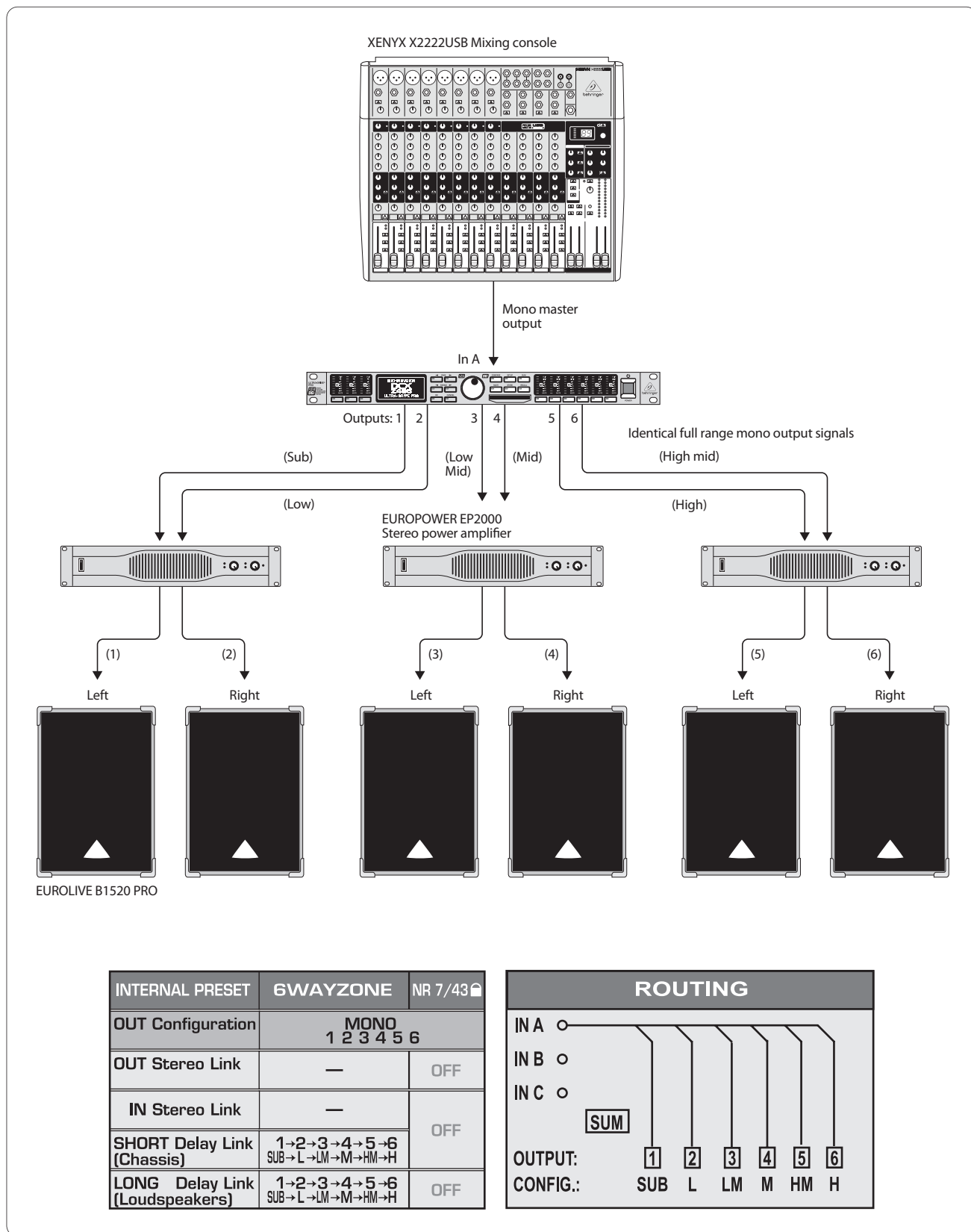
Afb. 6.7: Mono 6-weg "Zoning" (signaalverdeelmodus)
