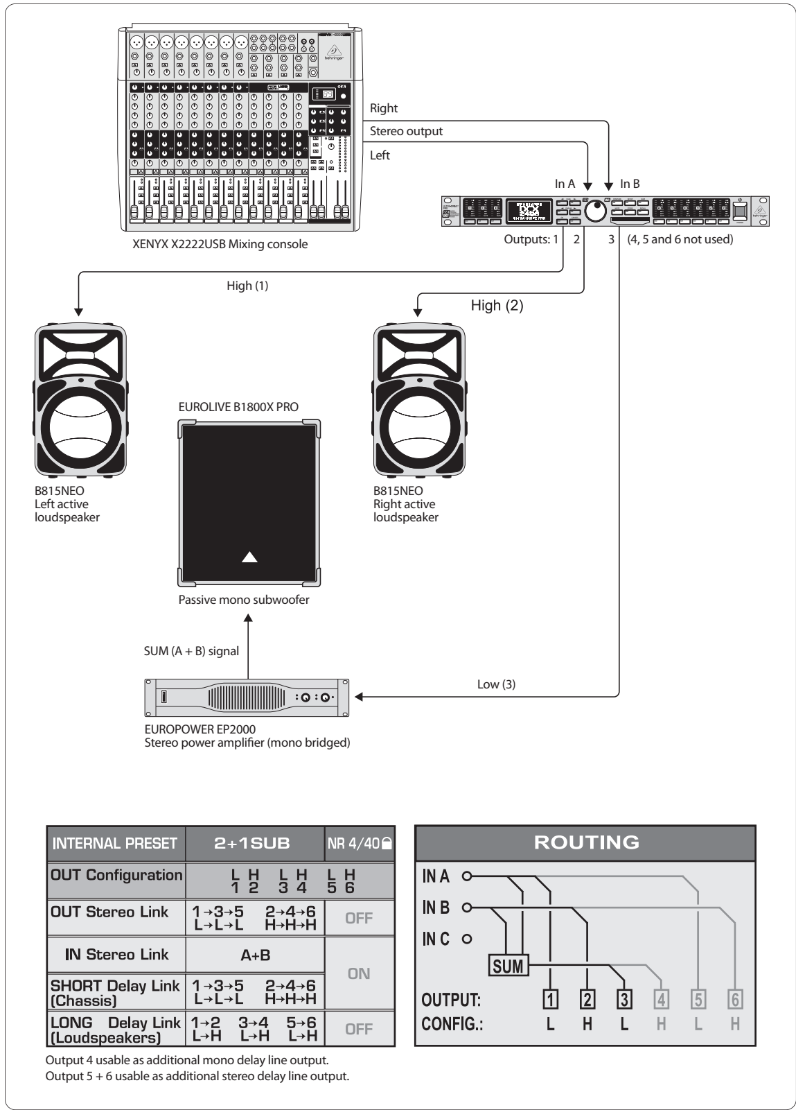
Afb. 6.4: Stereogebruik plus mono-subwoofer
