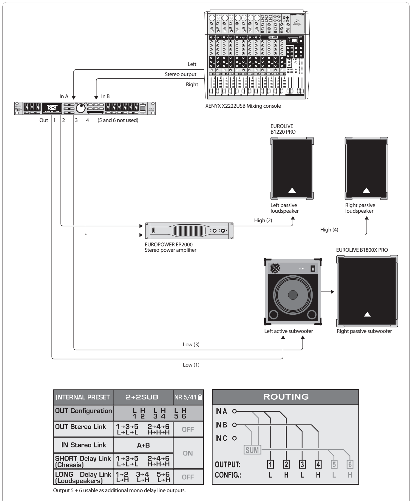
Afb. 6.5: Stereo gebruik plus 2 basboxen
