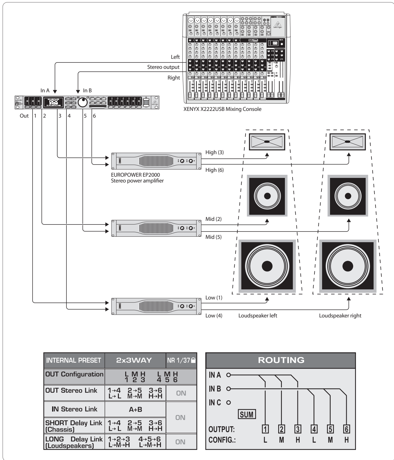
Afb. 6.1: Stereo 3-weg-gebruik
