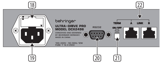
Afb. 2.4: Hoofdstroomaansluiting en de RS-232/RS-485-verbinding
