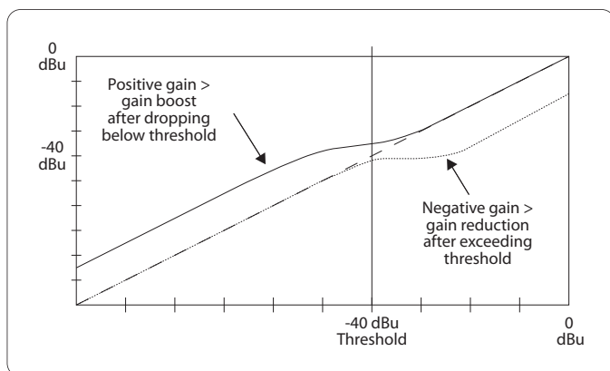
Afb. 4.36: Filtercurves bij over- c.q. overschrijden van de Threshold-waarde
