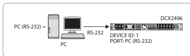
Afb. 4.26: De PC (RS-232)-modus
