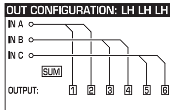
Afb. 4.2: Uitgangsconfiguraties
