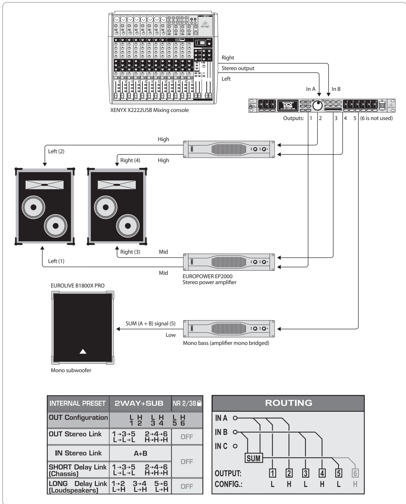
Afb. 6.2: Stereo 2-weg-gebruik plus subwoofer
