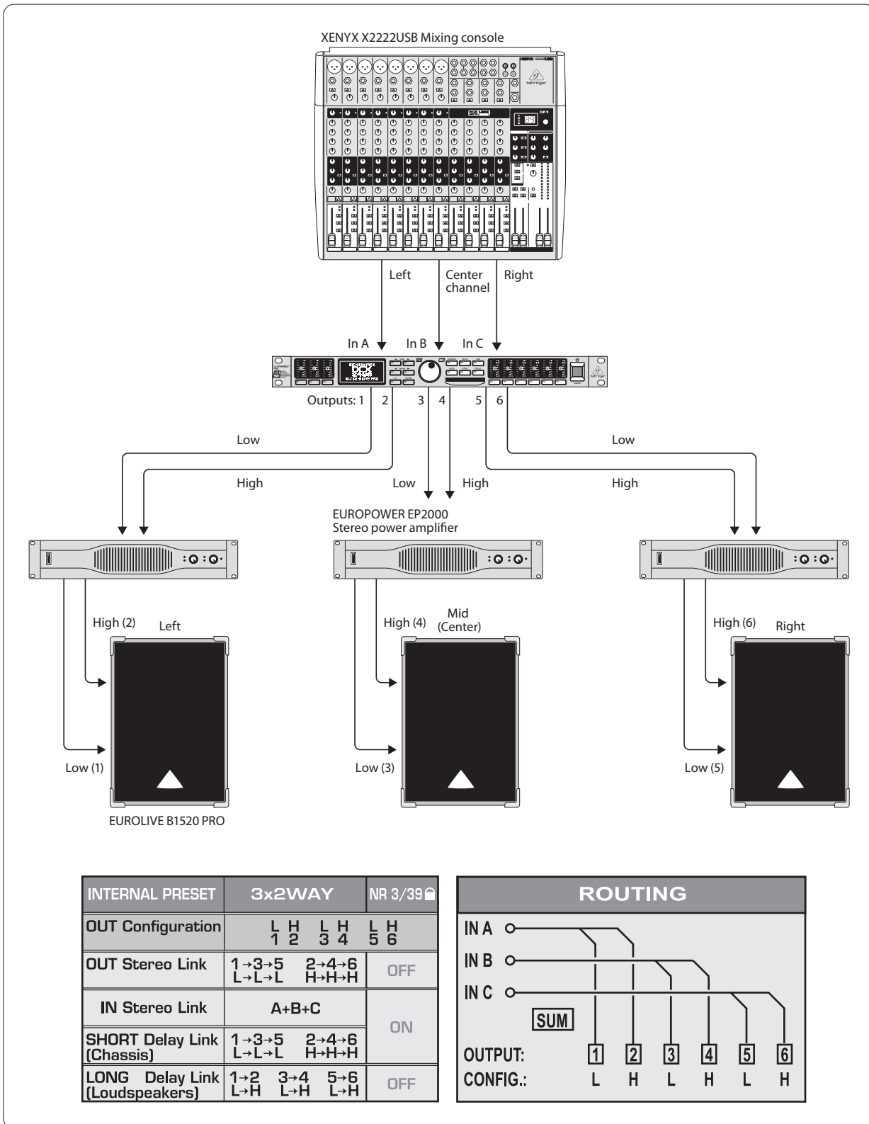
Afb. 6.3: 3x2-weg-gebruik [LCR/Triple Bi-Amping]
