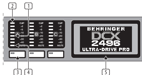
Afb. 2.1: Ingangs-LED's en display
