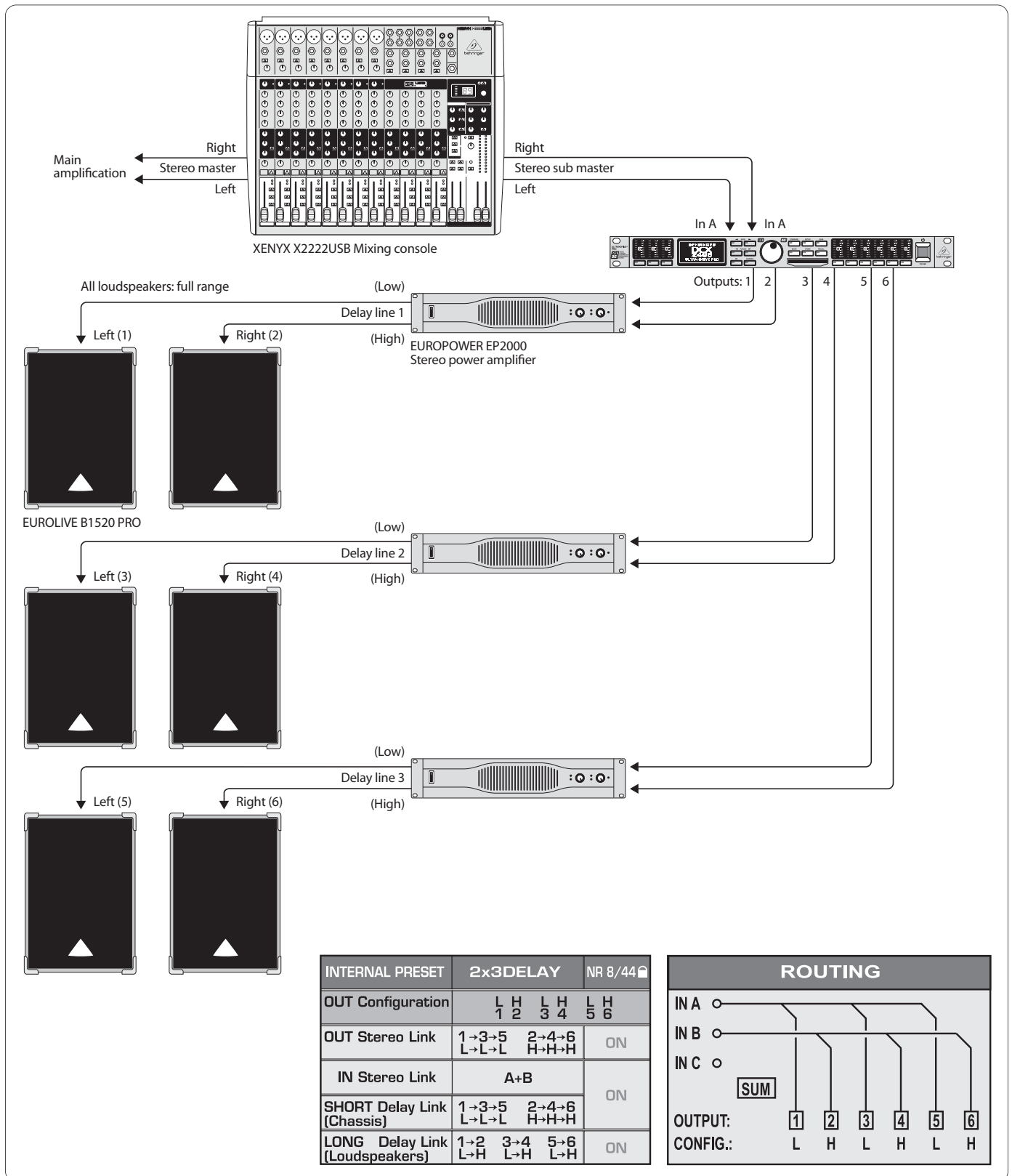
Afb. 6.8: Drievoudige Stereo Delay-Line
