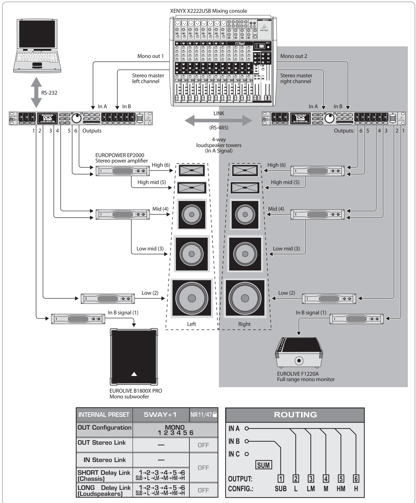
Afb. 6.11: 5-weg mono-gebruik plus 1 extra monosignaal (per stereokant)
