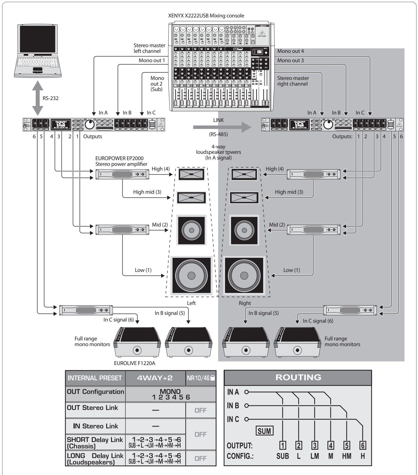
Afb. 6.10: 4-weg mono-gebruik plus 2 monitoren (per stereokant)
