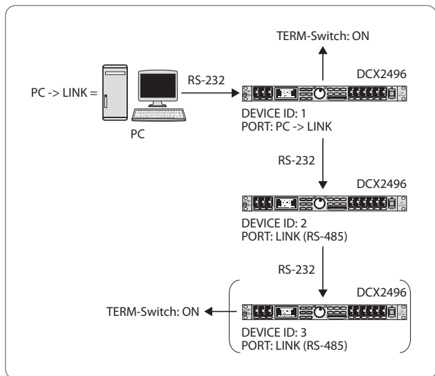
Afb. 4.30: De PC -> LINK-modus
